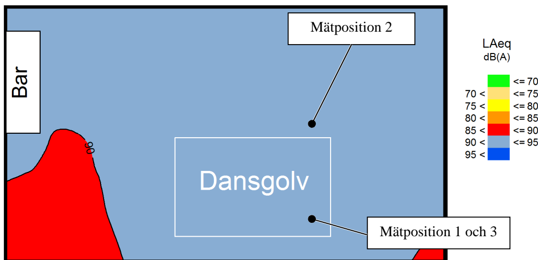
Figur 4 Ljudtrycksnivåer på en mindre nattklubb utritade som ljudnivåkonturer. Val av mätpunkter enligt avsnitt 5.2.1.
