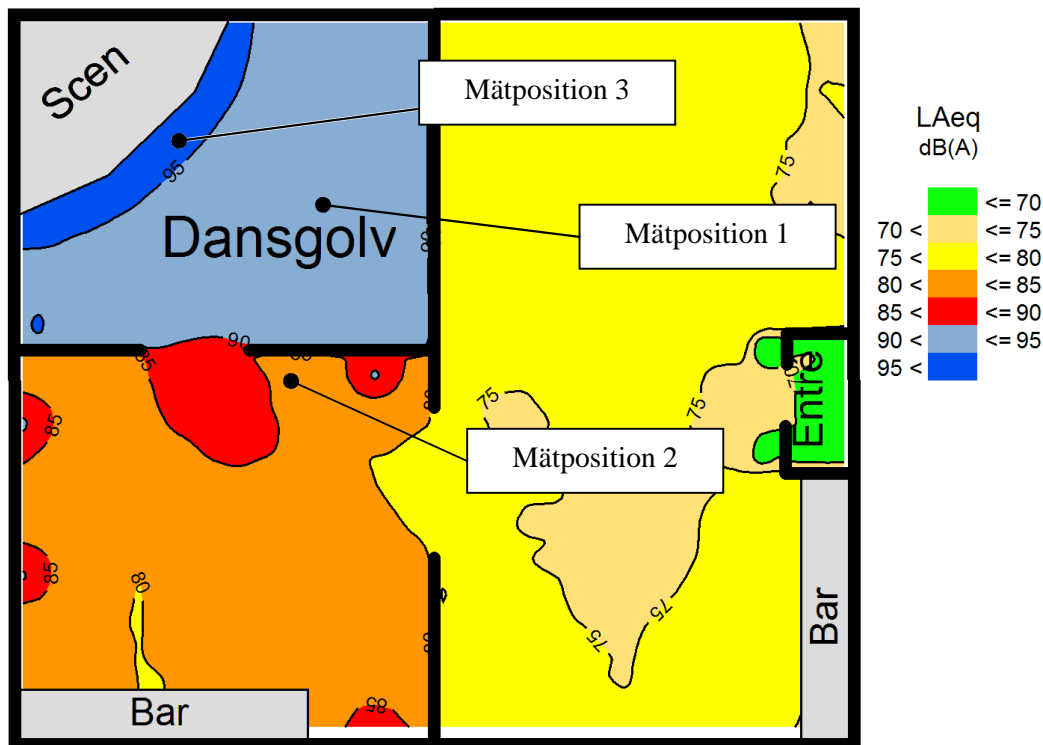
Figur 3 Ljudtrycksnivåer på en större nattklubb utritade som ljudnivåkonturer. Val av mätpunkter enligt avsnitt 5.2.1.
