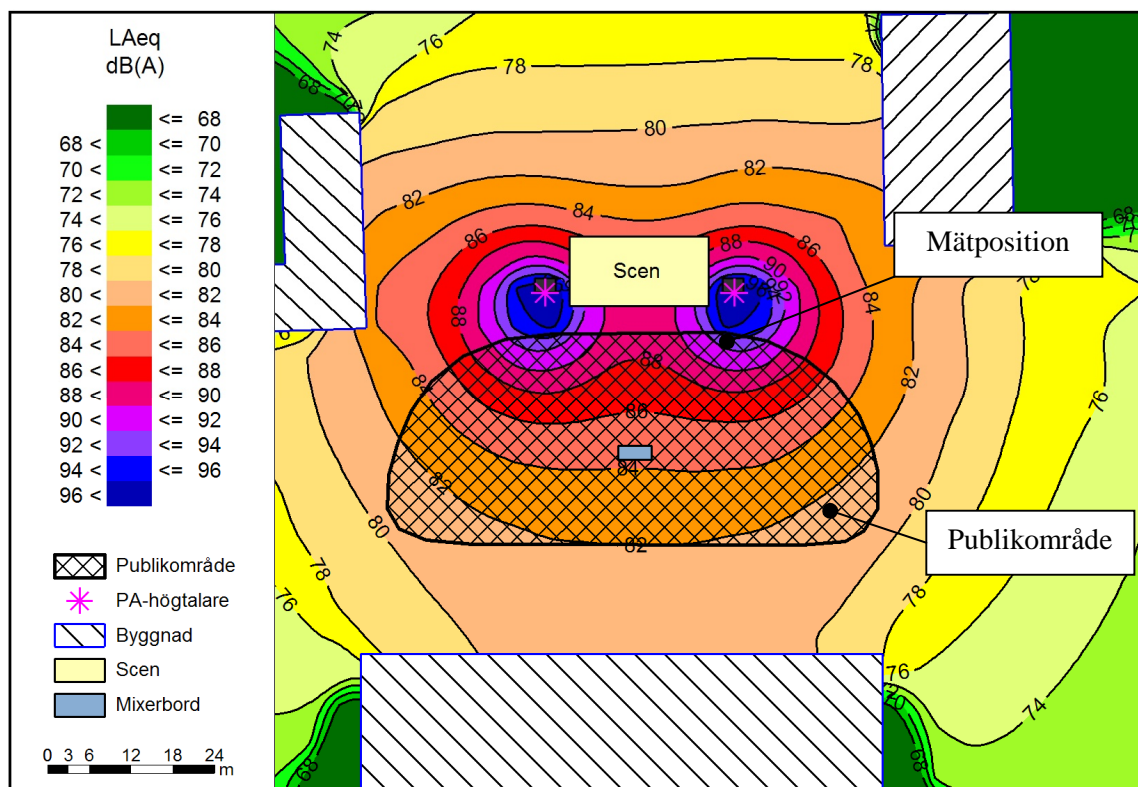
Figur 5 Ljudtrycksnivåer under första timmen vid en utomhuskonsert utritade som ljudnivåkonturer. Val av mätpunkt enligt avsnitt 5.1.1.
