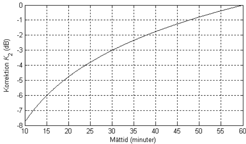
Figur 2 Korrektion K_2 vid avbruten mätning av L_{Aeq,1h} .
